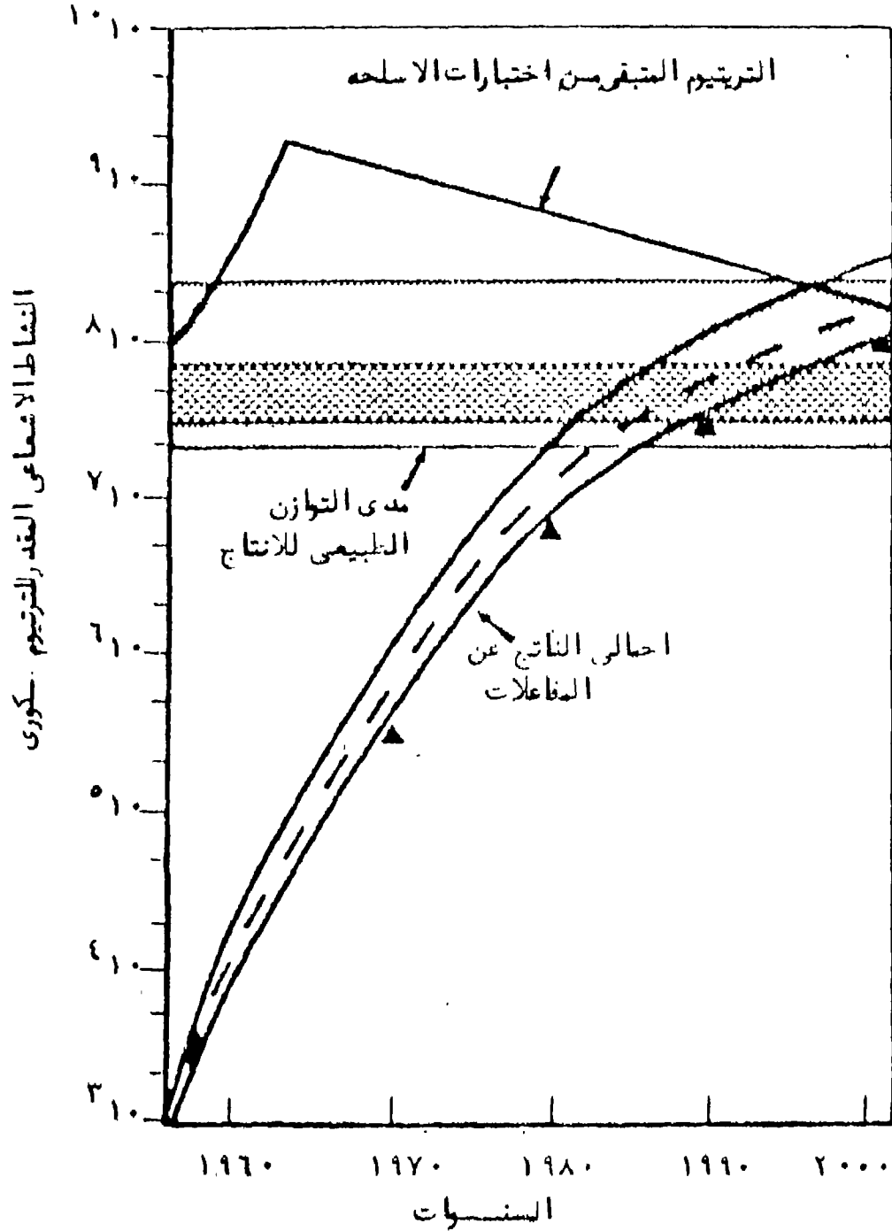
شكل (٢) : النشاط الإشعاعي للترتيوم في الجو من المصادر المختلفة.
